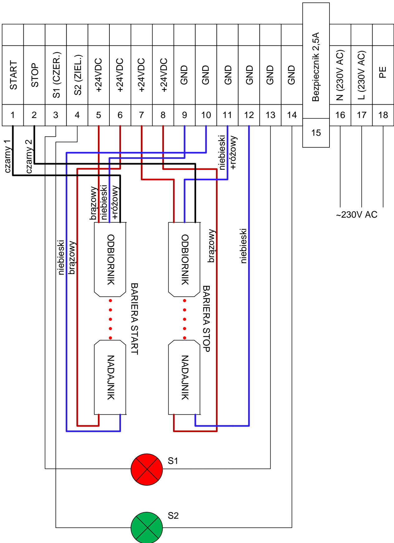
Rysunek 1. Typowy schemat połączeń sterownika pracującego w trybie SS-02 z sensorami fotoelektrycznymi firmy OMRON typu E3FC-TP11
